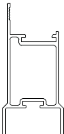
JA-MP318 0,401 Kg/m
