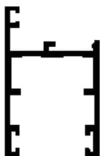
JA-25011 0,425 Kg/m
