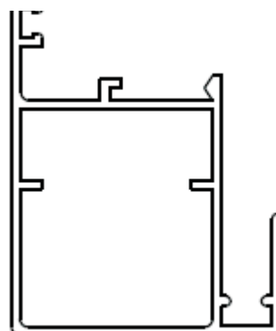
JA-25014 0,435 Kg/m
