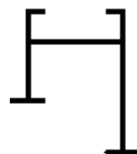
JA-DS205 0,130 Kg/m
